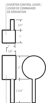
TEMPERATURE CONTROL LEVER / LEVIER DE CONTRÔLE DE LA TEMPÉRATURE
