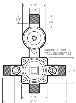
PRESSURE BALANCE VALVE / VANNES D'ÉQUILIBRAGE DE PRESSION Adjust screws to balance pressure in water lines / Adjuster les vis pour équilibrer la pression dans les conduits d'eau
