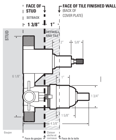
PRESSURE BALANCE VALVE / VANNES D'ÉQUILIBRAGE DE PRESSION Adjust screws to balance pressure in water lines / Adjuster les vis pour équilibrer la pression dans les conduits d'eau
