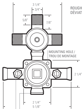
CAPPED / COUVERT Do not use valve / N'utilise pas la vanne PRESSURE BALANCE VALVE / VANNES D'ÉQUILIBRAGE DE PRESSION Adjust screws to balance pressure in water lines / Adjuster les vis pour équilibrer la pression dans les conduits d'eau
